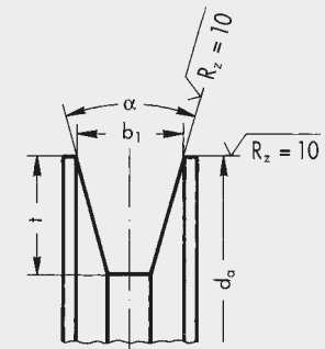
Polea de medición para correas trapeciales estrechas de alto rendimiento norma USA RMA/MPTA
