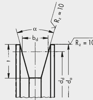
Polea de medición para correas trapeciales estrechas de alto rendimiento DIN 7753 parte 1 y correas trapeciales clásicas DIN 2215
