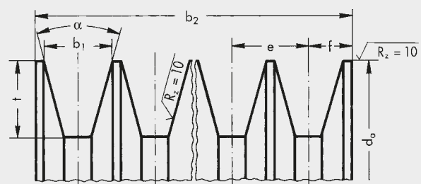
Polea de medición para correas múltiples
