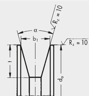
Polea de medición para correas hexagonales
